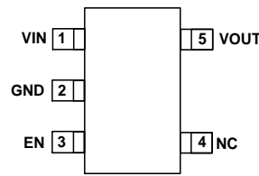
SOT25
