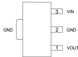
SOT89
