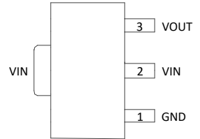
SOT89
