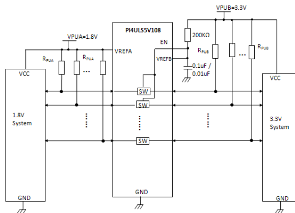
PI4ULS5V108
