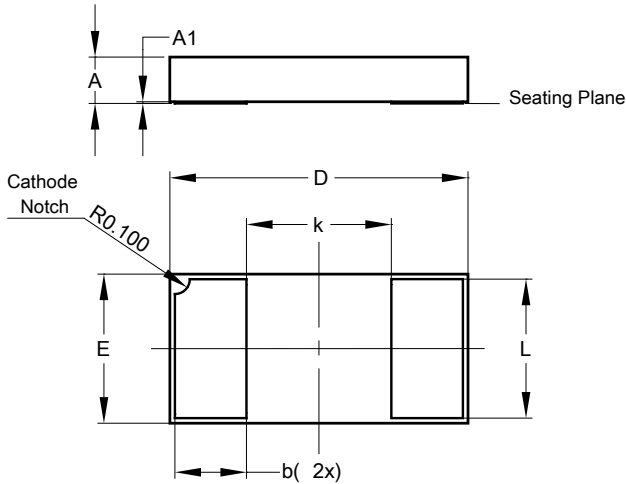
X2-WLB2010-2
