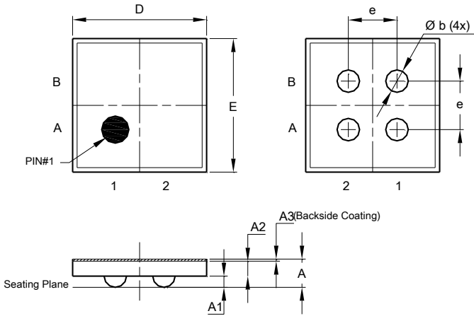
X1-WLB1818-4
