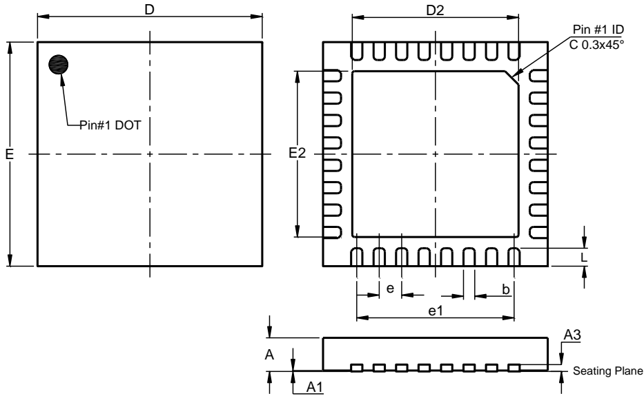
W-QFN5050-32
