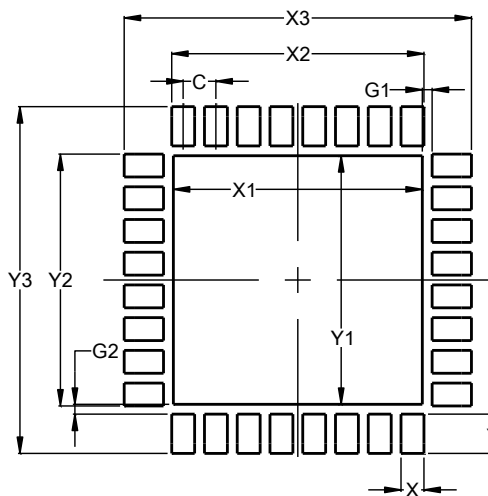
W-QFN5050-32
