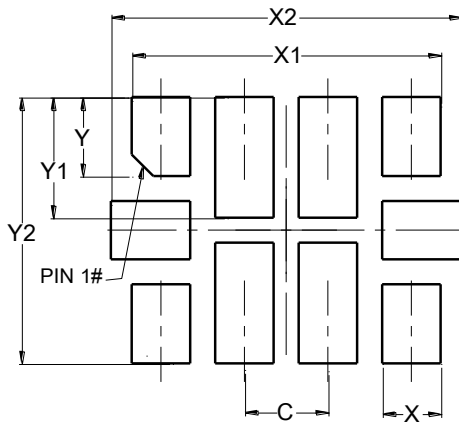
W-QFN1520-10
