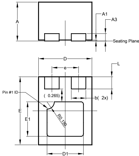
W-DFN1114-3
