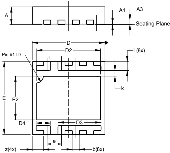
V-DFN3333-8
