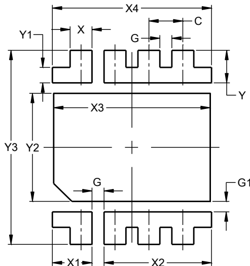
V-DFN3333-8
