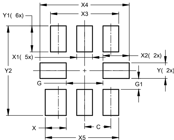
U-FLGA1616-8
