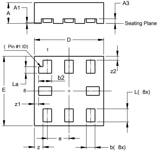
U-FLGA1616-8
