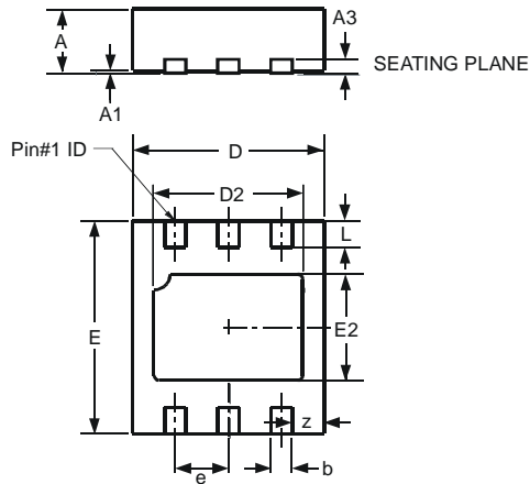
U-DFN2018-6
