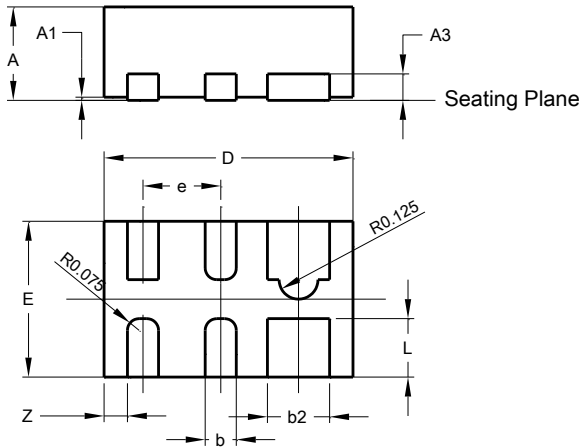
U-DFN1610-6
