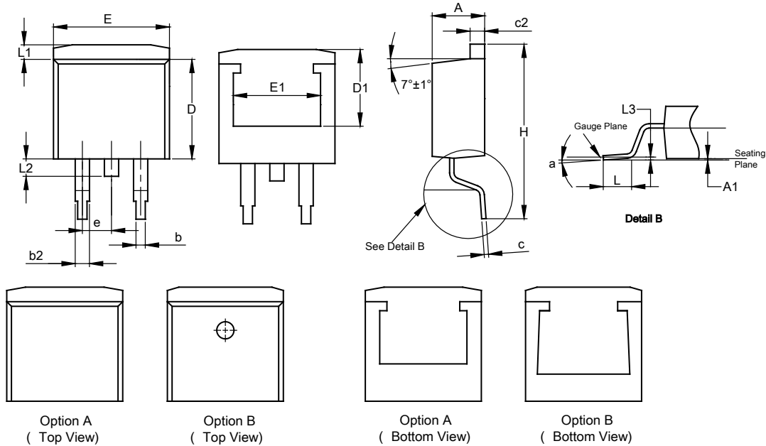
TO263AB (Standard)
