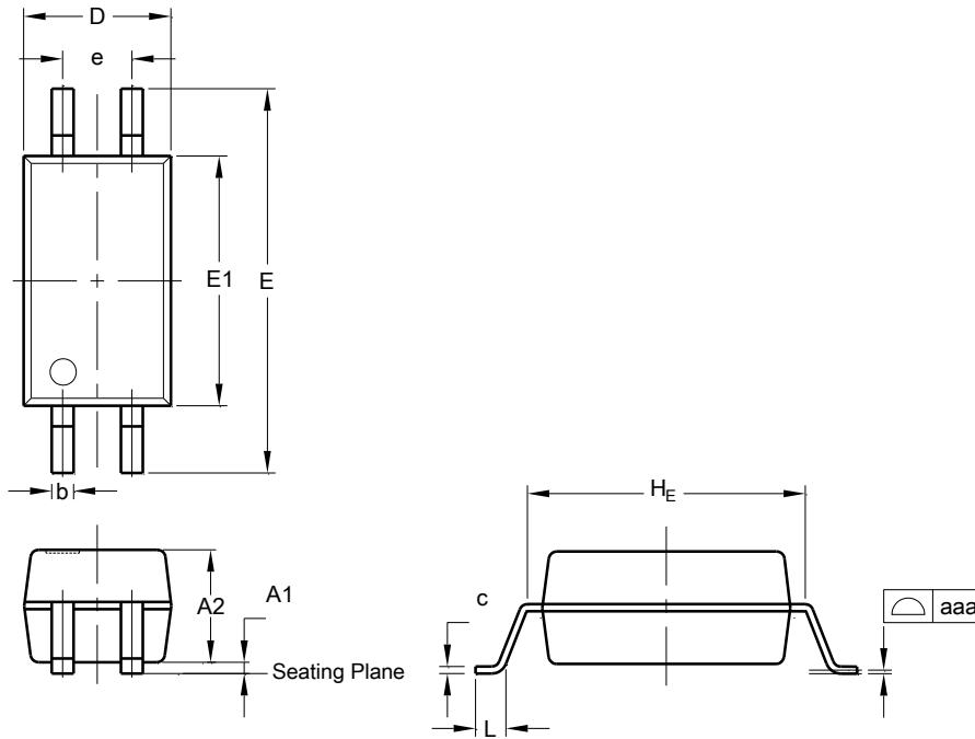
SSOP-4
