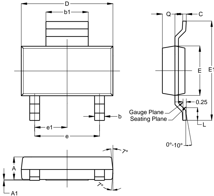
SOT223-3
