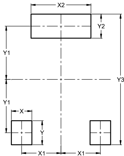
SOT223-3
