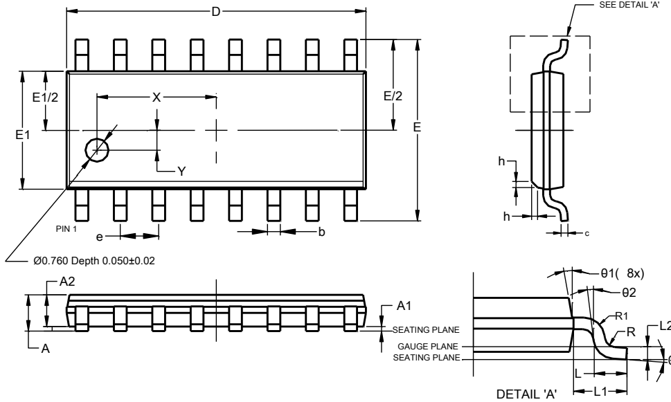
SO-16
