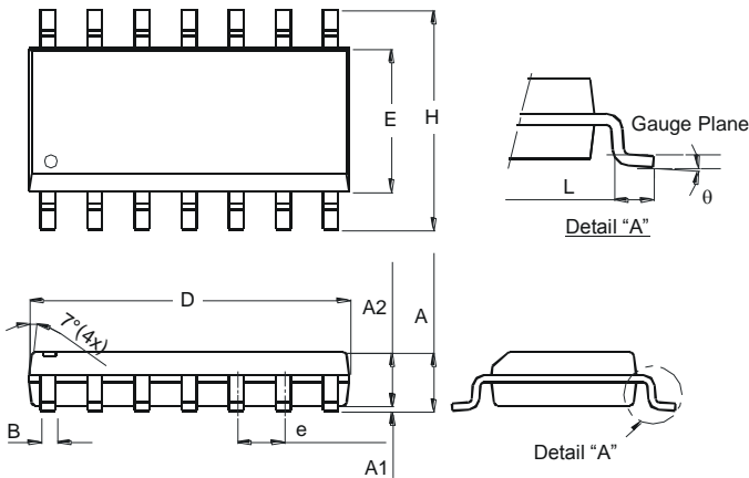
SO-14
