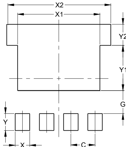
PowerDI8080-5
