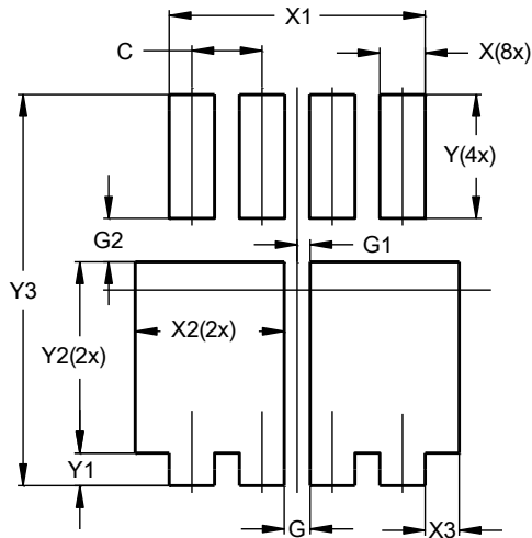
PowerDI3333-8 (Type E)
