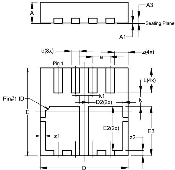
PowerDI3333-8 (Type E)
