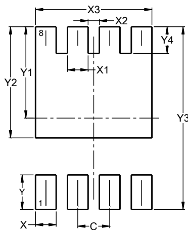
PowerDI3333-8 (SWP)
