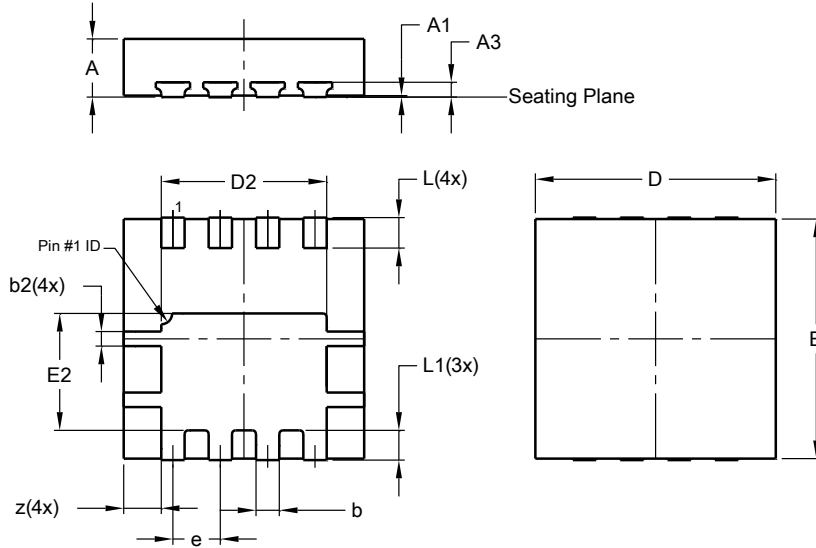
PowerDI3333-8 (SWP)
