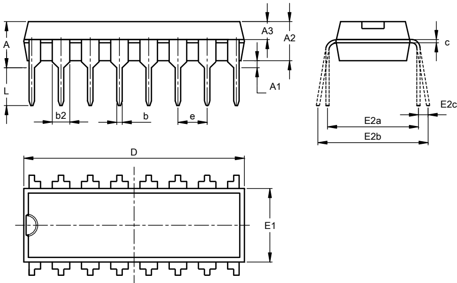
PDIP-16
