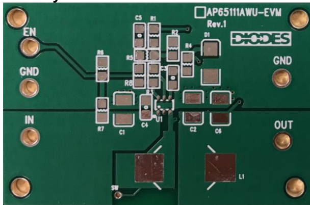
Top Layer
