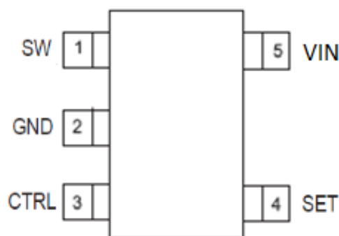
TSOT25 package
