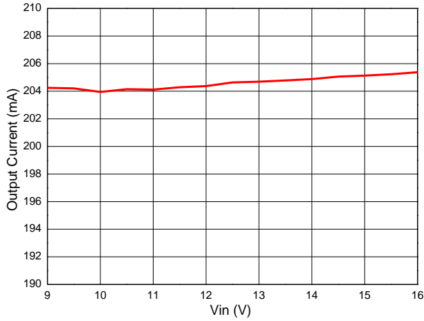
Output Current vs. Vin
