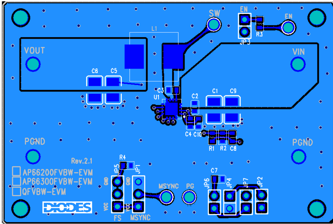
Figure 3. AP66300QFVBW-EVM – Top Layer
