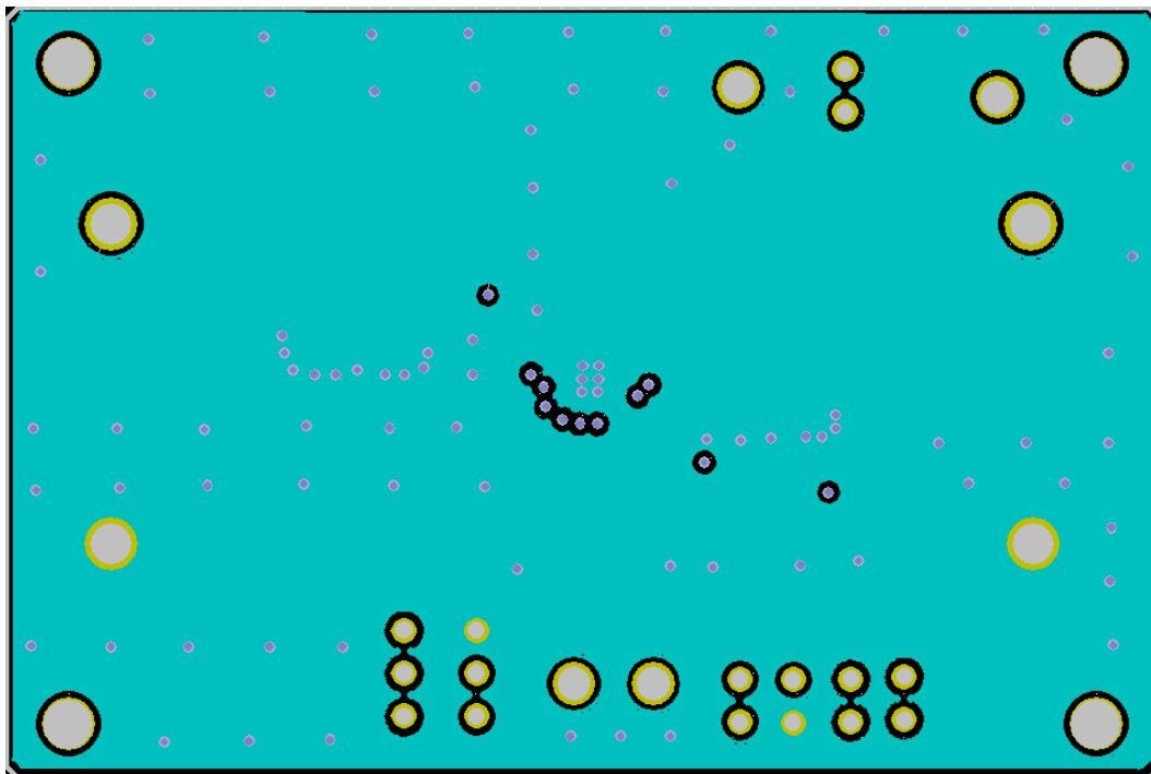
Figure 4. AP66300QFVBW-EVM – Layer 2
