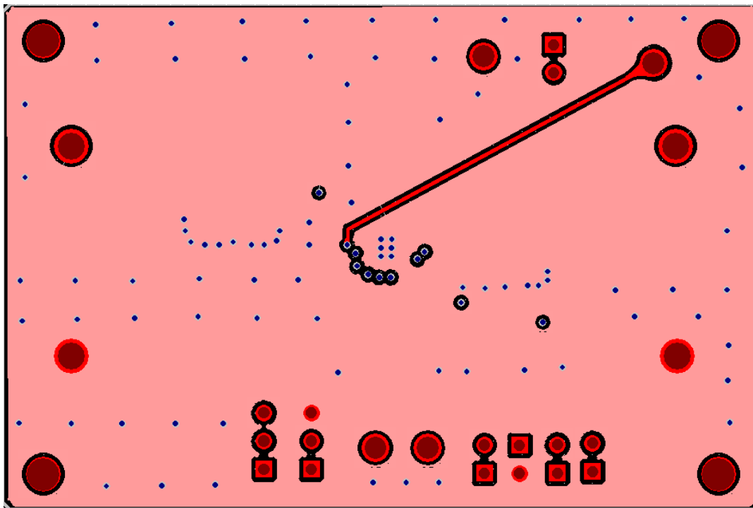
Figure 6. AP66300QFVBW-EVM – Bottom Layer
